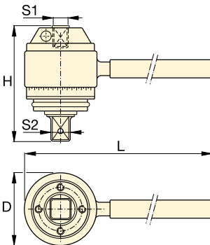
Abstützhebel-Typ 1)
